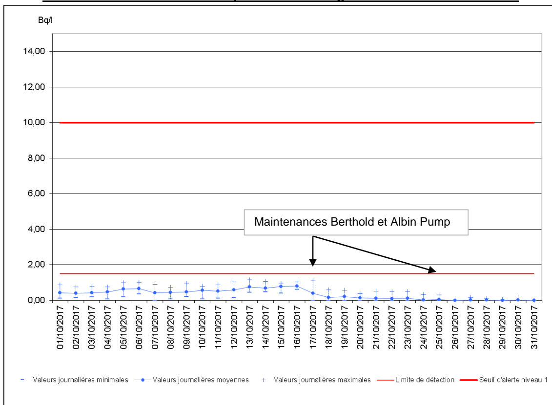
Evolution des activités volumiques de la voie « gamma total » - Octobre 2017
